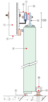
C트랙 / 하부레일
