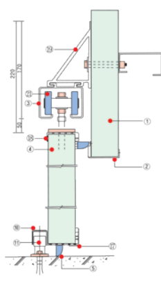
M트랙 / 하부레일
