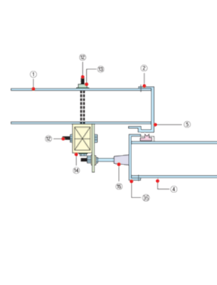
하부스톱바 구성도
